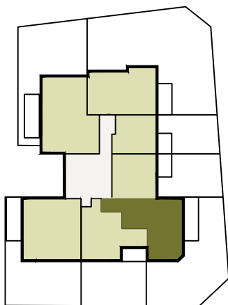
KARTA MIESZKANIA M24 1:100
